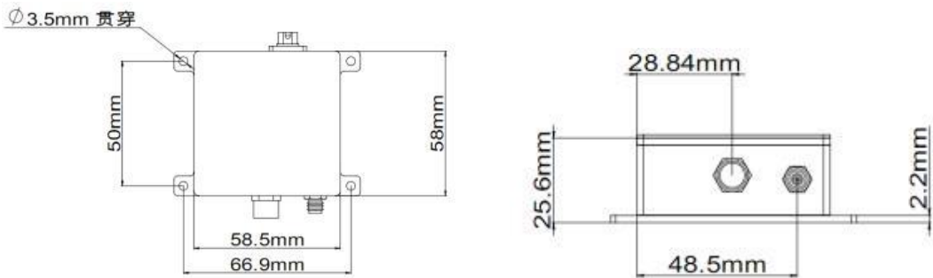
图 4-1 APD 探测器模块机械尺寸图
